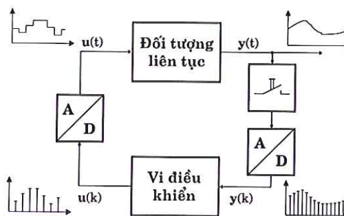
H. 1 Cấu trúc của hệ thống điều khiển số
